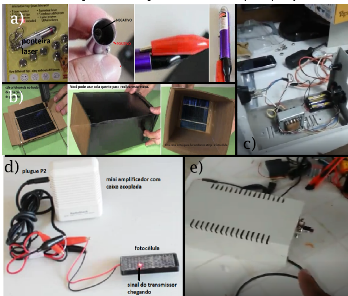
Figura 12 – Montagem do transmissor AM para aplicação
